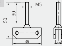
磁块架
