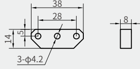
磁块
